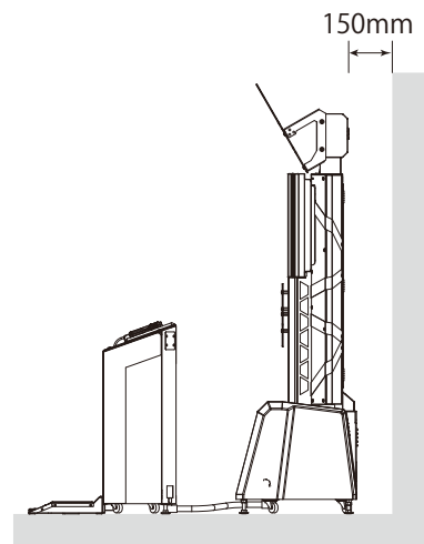
FIG. 6-3e Ventilation Space
